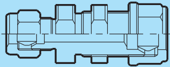
RBUH 異径バルクヘッド ユニオン REDUCING BULKHEAD UNION
