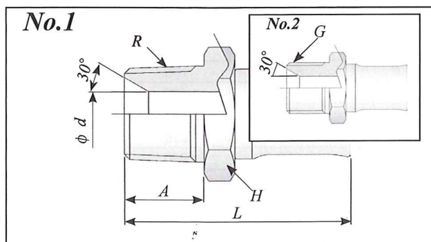
No.1・No.2 金具 材質：鉄/ステンレス
