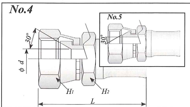
No.4 No.5 金具 材質：鉄/ステンレス
