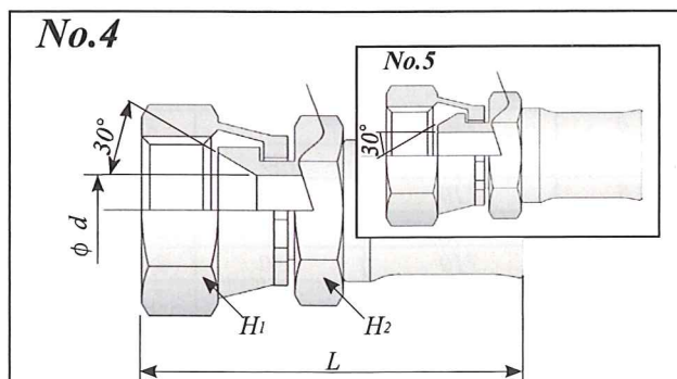
No.4 No.5 金具 材質：鉄/ステンレス
