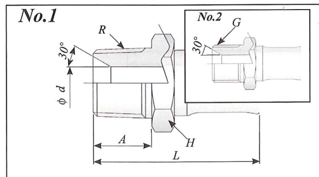
No.1・No.2 金具 材質：鉄/ステンレス
